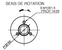
DETAIL DE LA POULIE (A) ECHELLE 1/3
